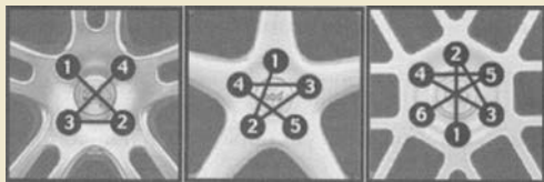
Схемы затягивания/отвинчивания гаек или болтов
